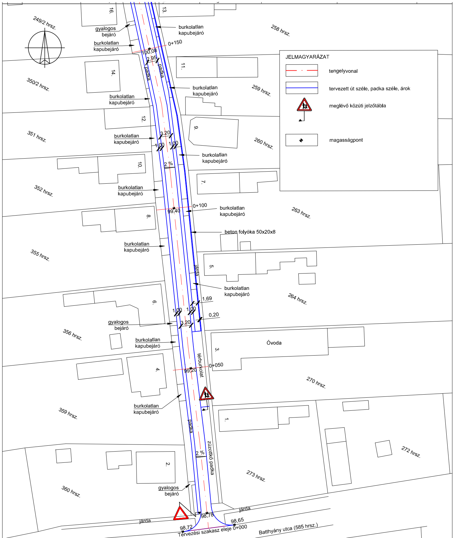
HELYSÍNRAJZ M 1:500
